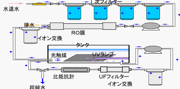
超純水製造装置構成図
