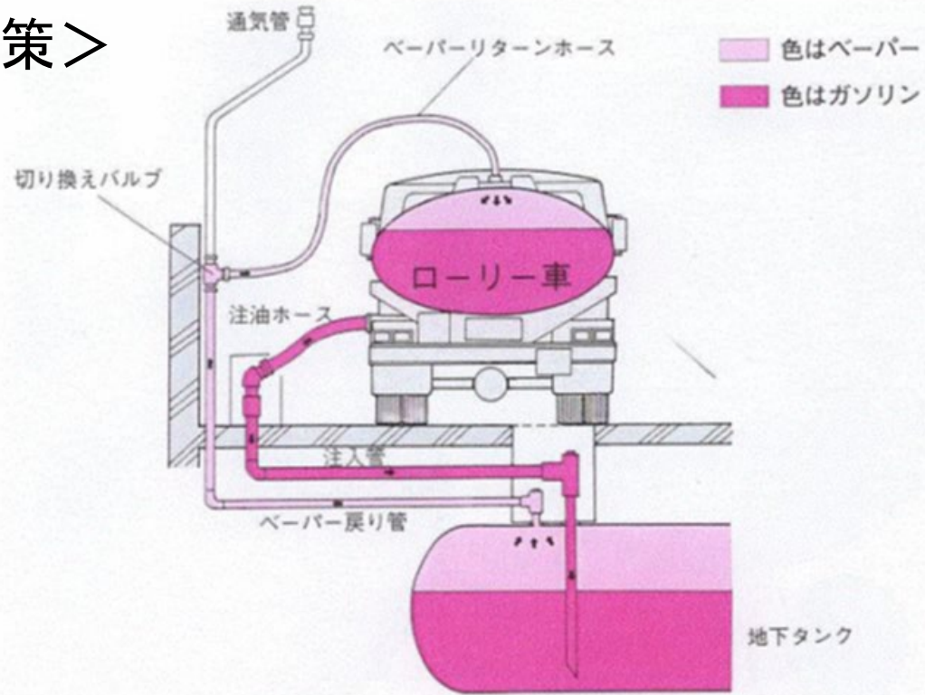
図. ベーパーリターン装置
