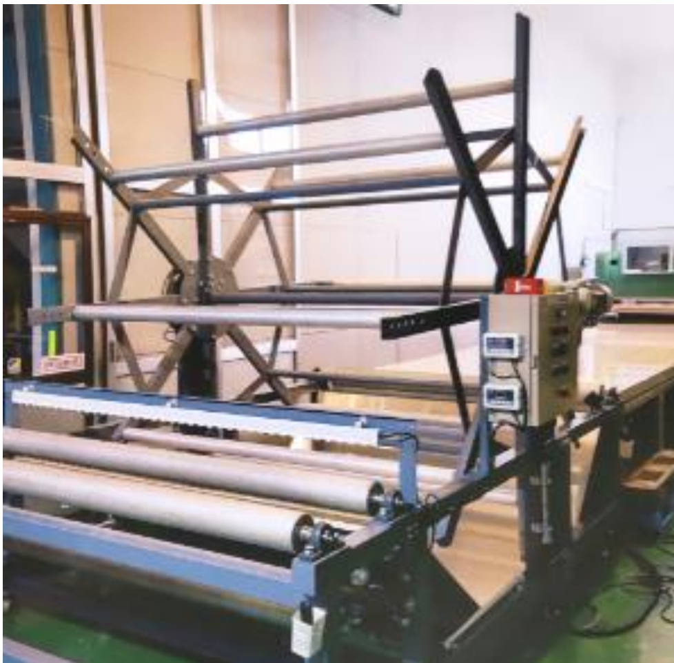
不織布スリッター付大型自動延反機
